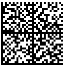
Esempio codice
